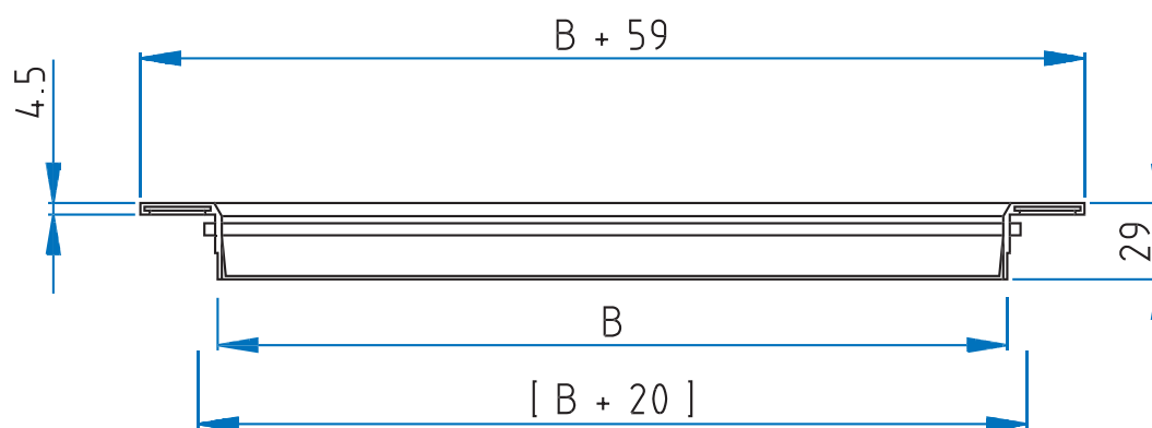
AG-100 NE (waagrechte, einzeln einstellbare Tropflamellen)
