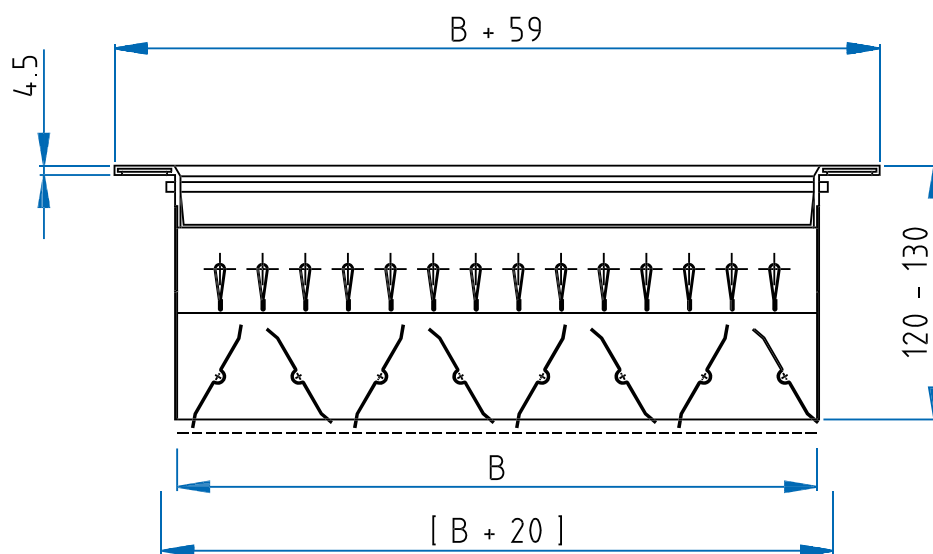
AG-230 AG-200 mit MKL-2 (gekuppelte gegenläufige Mengenregulierung)
