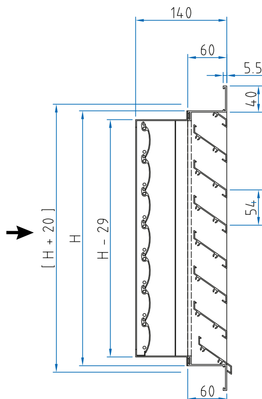
ALG AL/JK AL-V Lamellen nach vorne öffnend
