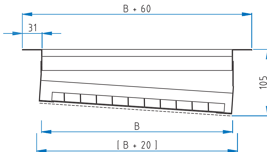
G-150 R G-100 R mit SO-A (schräger Schlitzschieber-Aufsatz)
