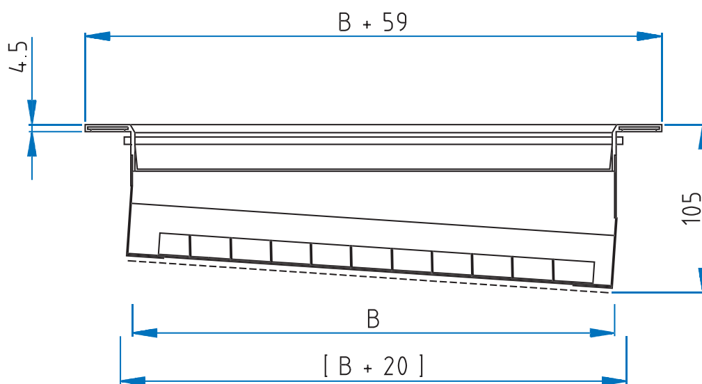
AG-150 NE AG-100 NE mit SO-A (schräger Schlitzschieber-Aufsatz)
