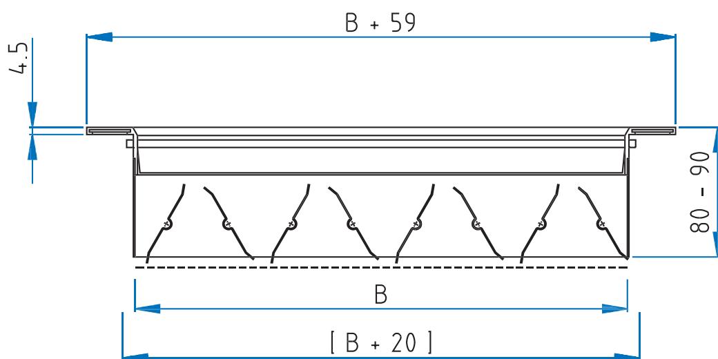
AG-130 AG-100 mit MKL-2 (gekuppelte gegenläufige Mengenregulierung)
