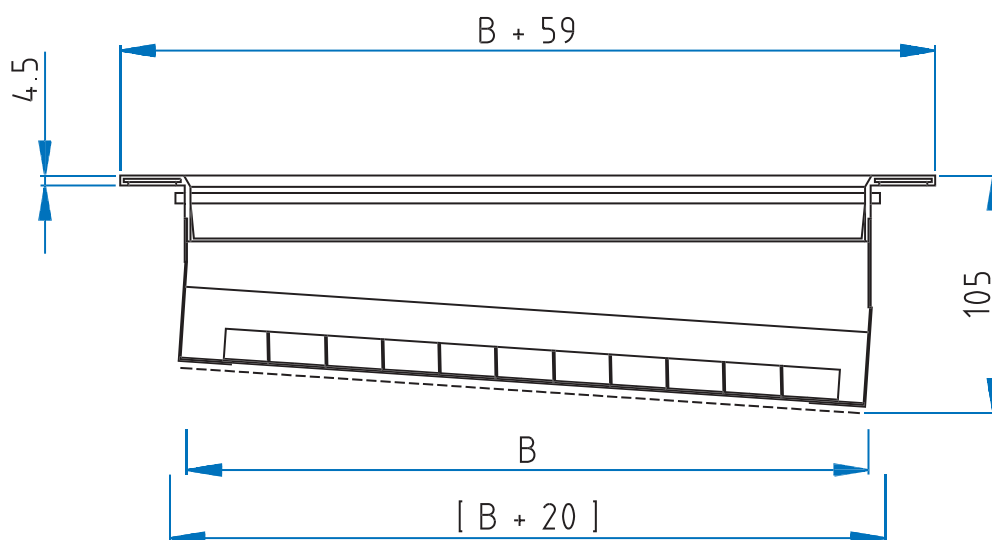
AG-150 AG-100 mit SO-A (schräger Schlitzschieber-Aufsatz)
