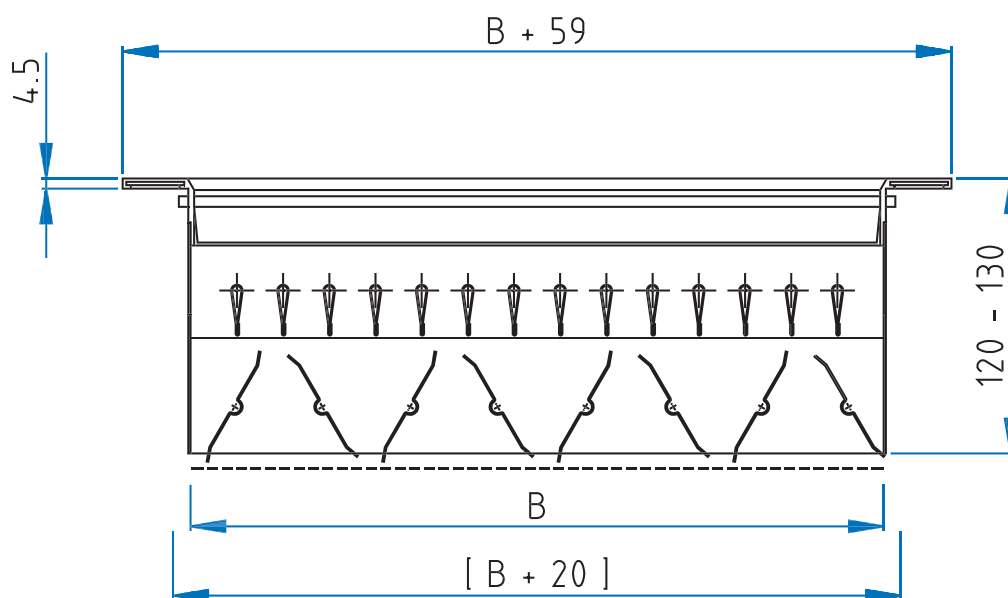
AG-230 NE AG-200 NE mit MKL-2 (gekuppelte gegenläufige Mengenregulierung)
