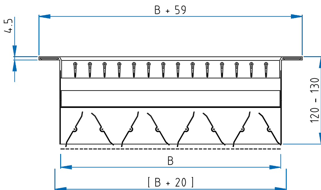
AG-530 AG-500 mit MKL-2 (gekuppelte gegenläufige Mengenregulierung)
