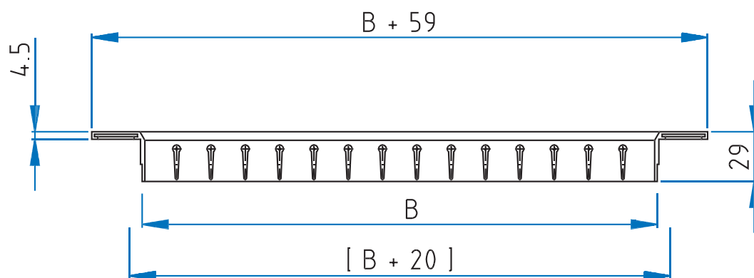
AG-600 NE (vorne senkrechte, einzeln einstellbare Tropflamellen)
