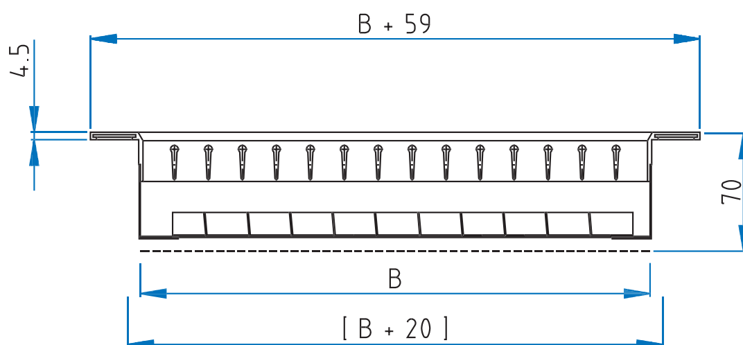
AG-640 NE AG-600 NE mit SO (Schlitzschieber)
