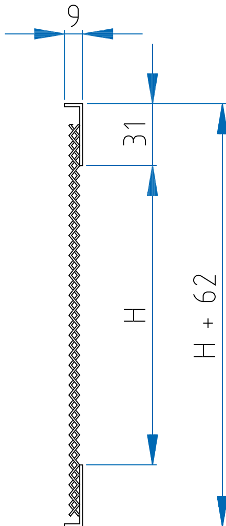
BG-B Abdeckgitter mit Steckmetall
