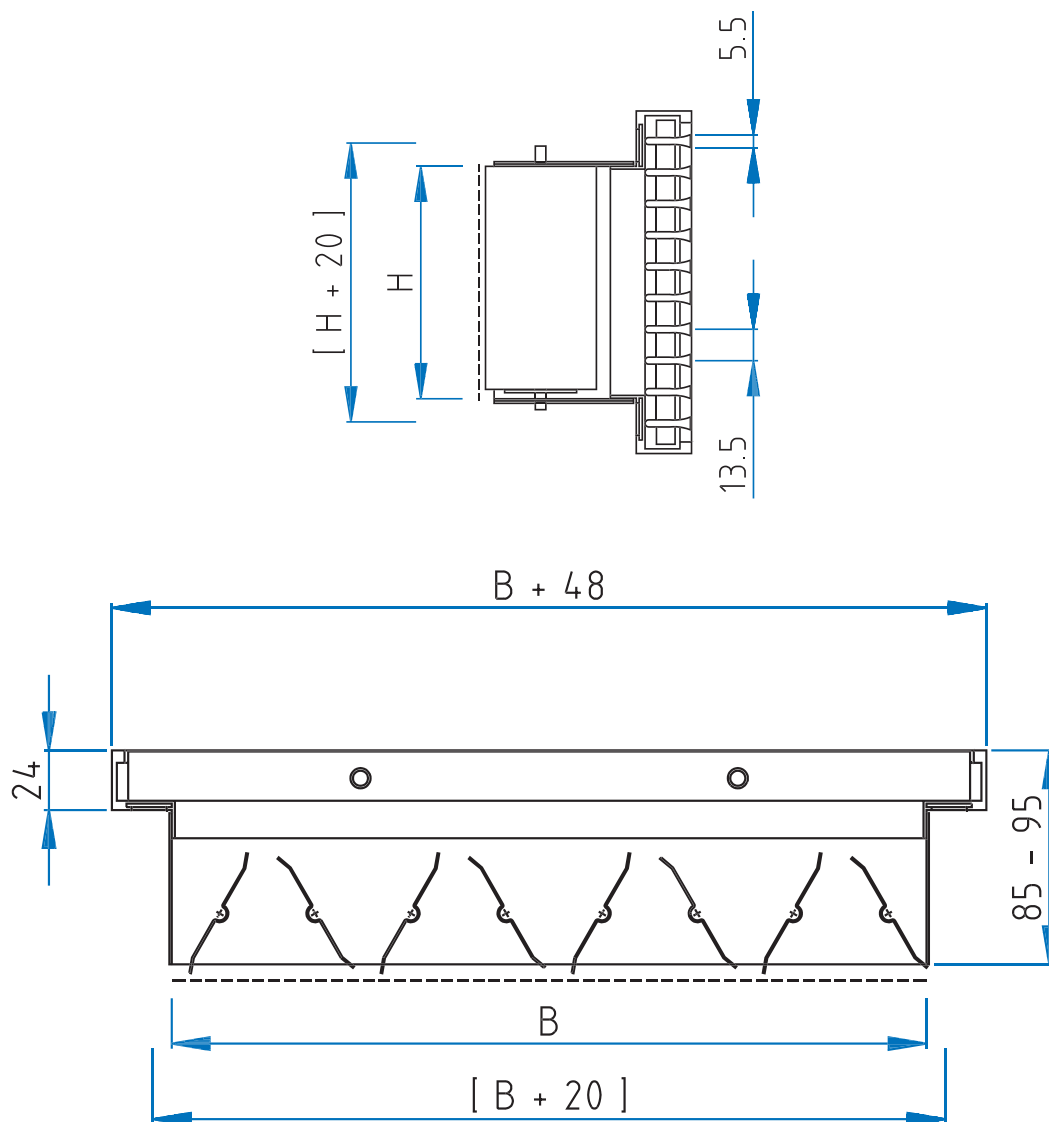
F-130 F-100 mit MKL-2 (gekuppelte gegenläufige Mengenregulierung)
