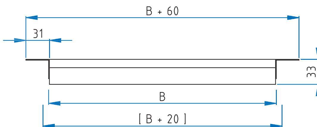
G-100 R (waagrechte, einzeln einstellbare Tropflamellen)
