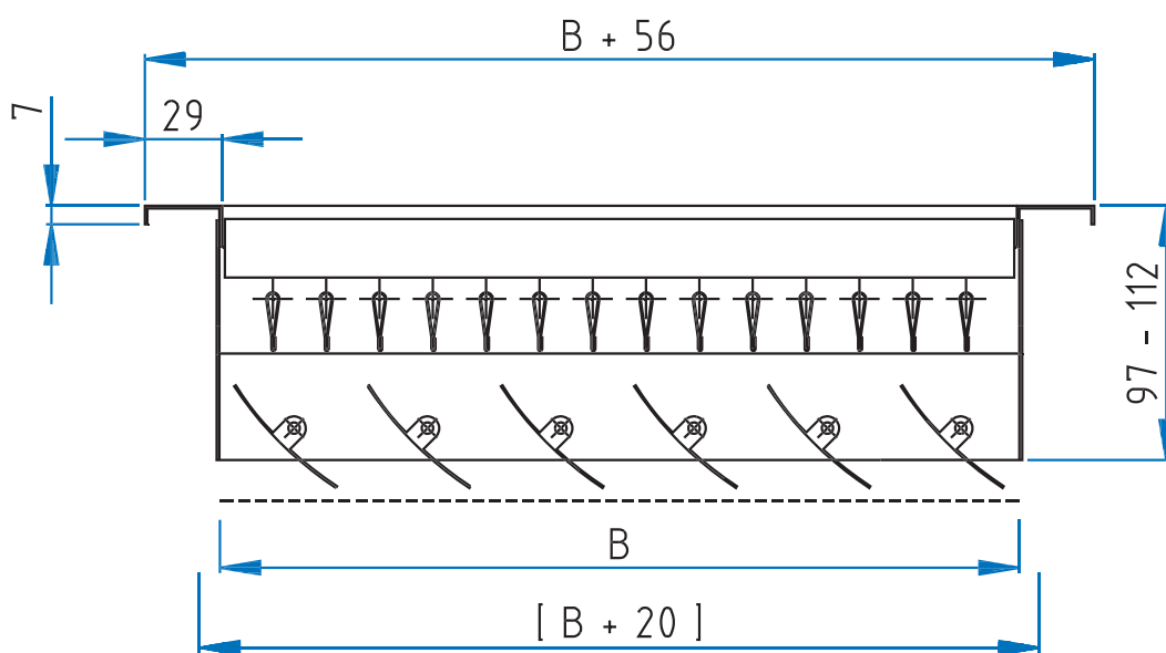
G-220 G-200 mit MKL-1 (einzeln einstellbare Schöpflamellen)
