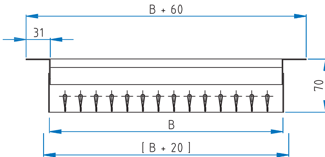
G-200 R (vorne waagrechte, und hinten senkrechte einzeln einstellbare Tropflamellen)
