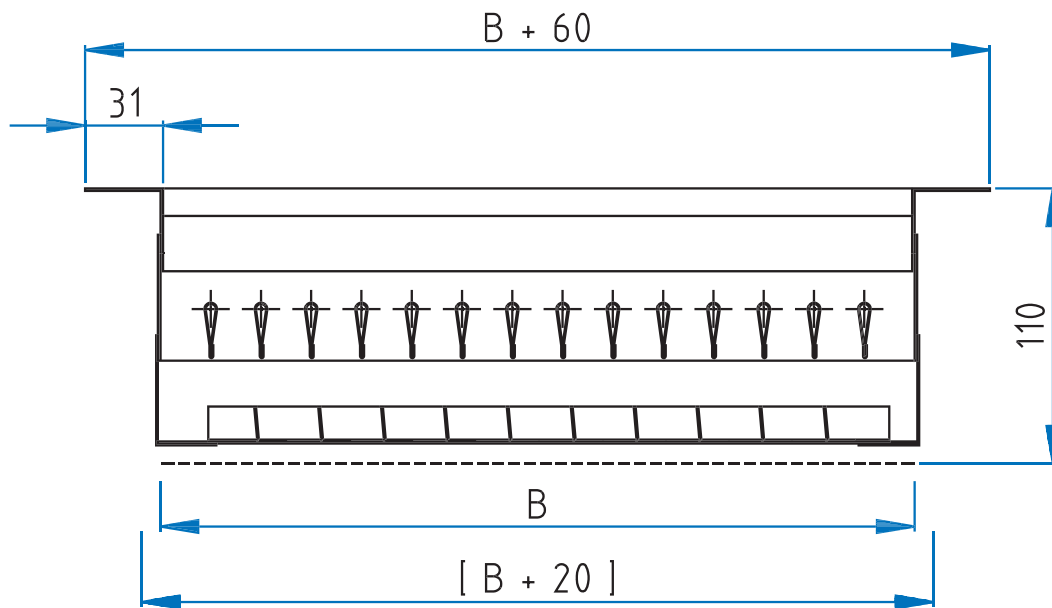
G-240 R G-200 R mit SO (Schlitzschieber)
