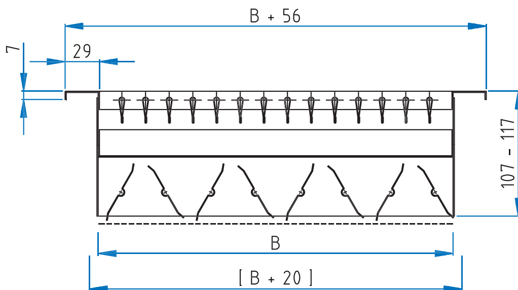
G-530 G-500 mit MKL-2 (gekuppelte gegenläufige Mengenregulierung)
