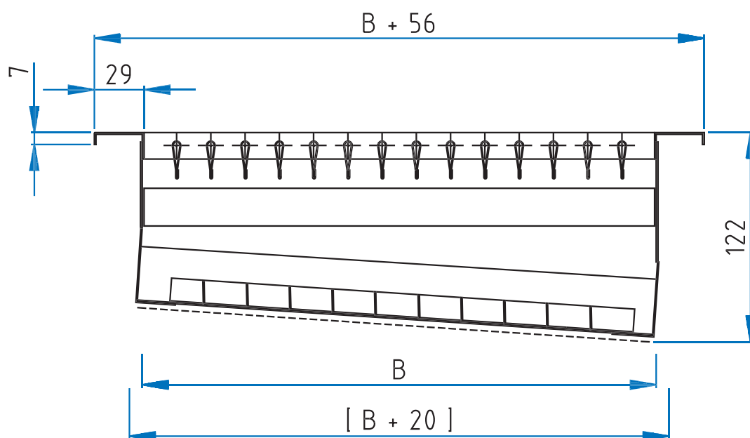
G-550 G-500 mit SO-A (schräger Schlitzschieber-Aufsatz)
