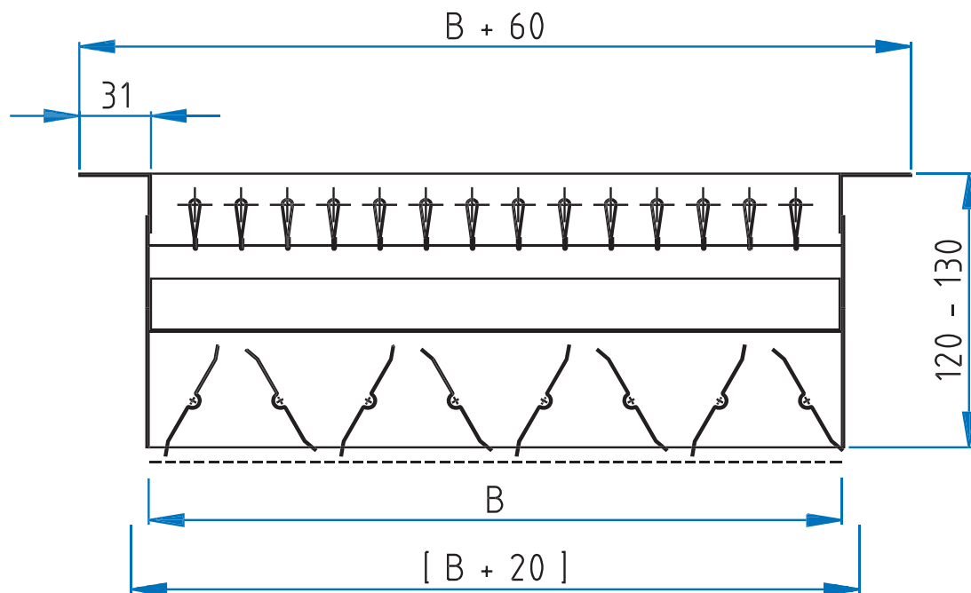
G-530 R G-500 R mit MKL-2 (gekoppelte gegenläufige Mengenregulierung)
