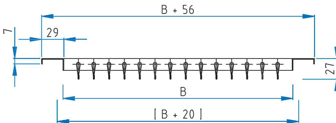
G-600 (vorne senkrechte, einzeln einstellbare Troplamellen)
