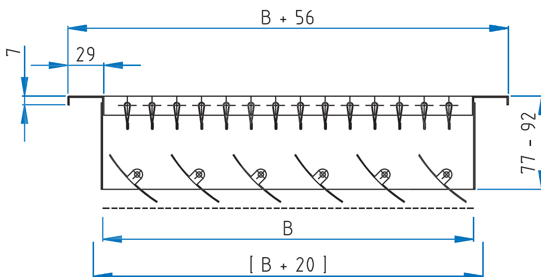
G-620 G-600 mit MKL-1 (einzeln einstellbare Schöpflamellen)
