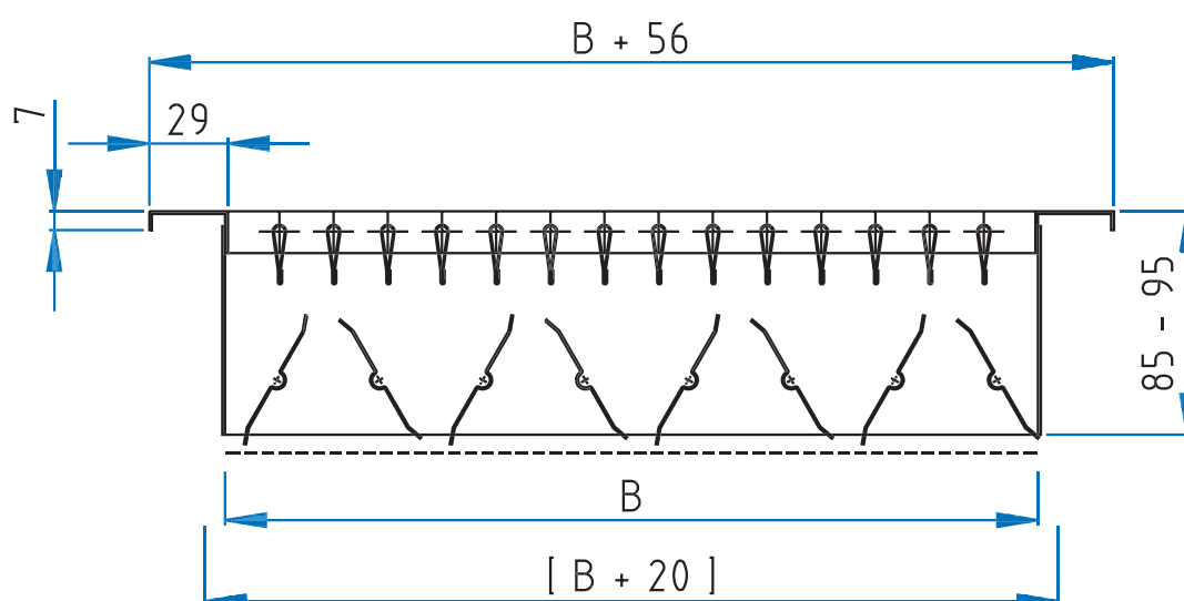
G-630 G-600 mit MKL-2 (gekuppelte gegenläufige Mengenregulierung)
