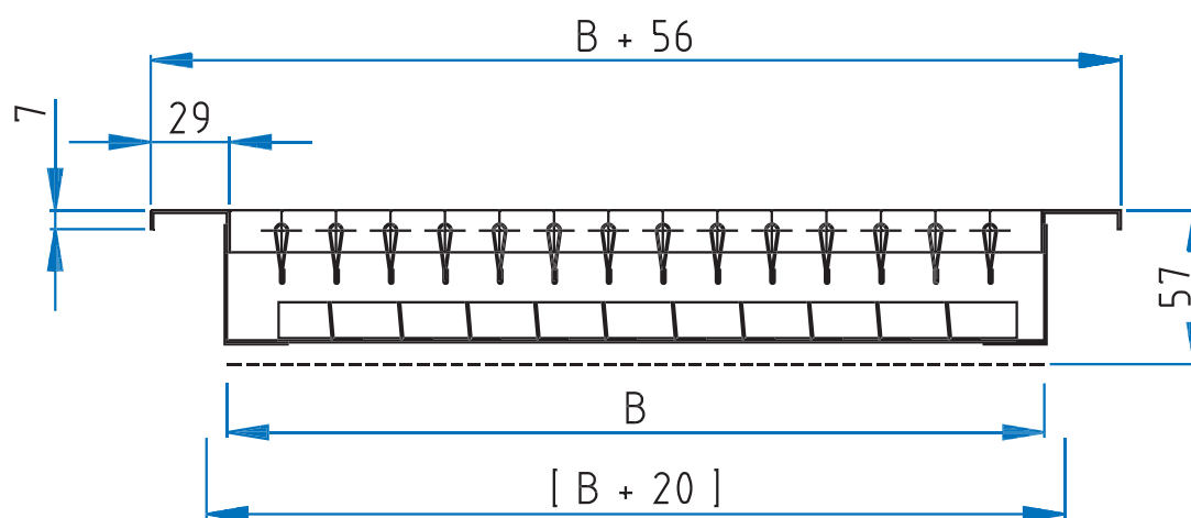
G-640 G-600 mit SO (Schlitzschieber)
