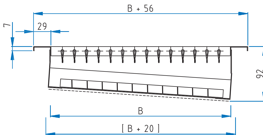
G-650 G-600 mit SO-A (schräger Schlitzschieber-Aufsatz)
