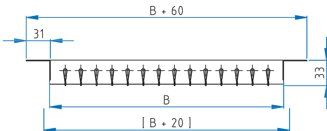
G-600 R (vorne senkrechte, einzeln einstellbare Tropflamellen)
