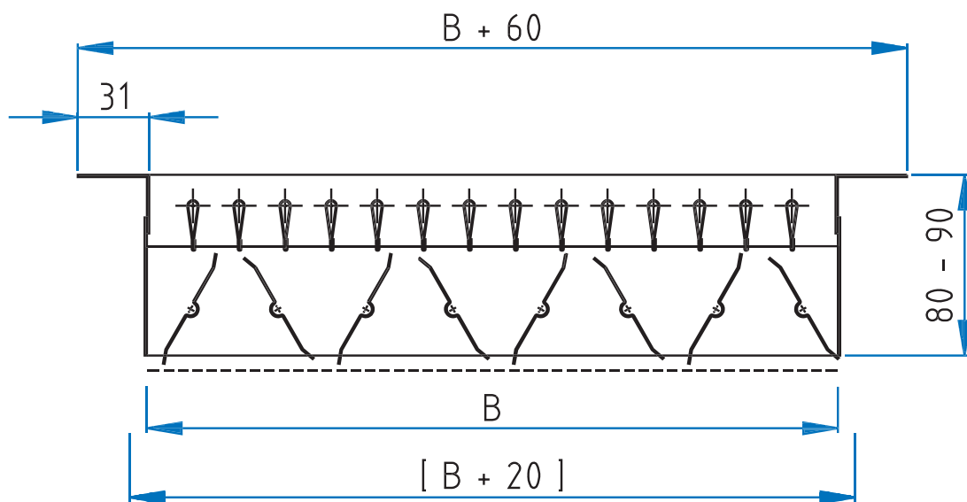
G-630 R G-600 R mit MKL-2 (gekoppelte gegenläufige Mengenregulierung)
