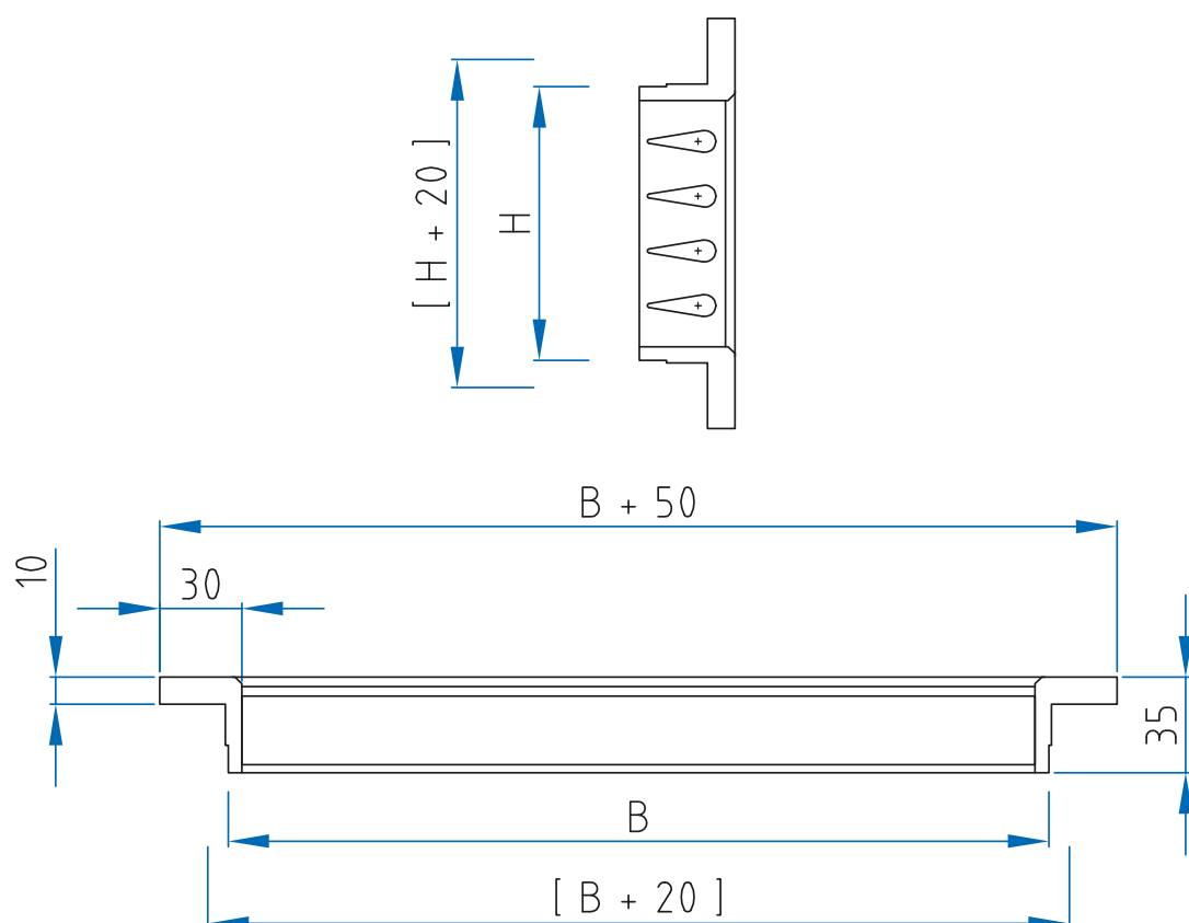
HG-100 (waagrechte, einzeln einstellbare Tropflamellen)
