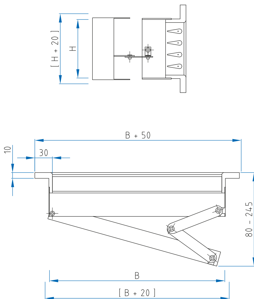
HG-110 HG-100 mit Z (einstellbare Schöpfzunge)
