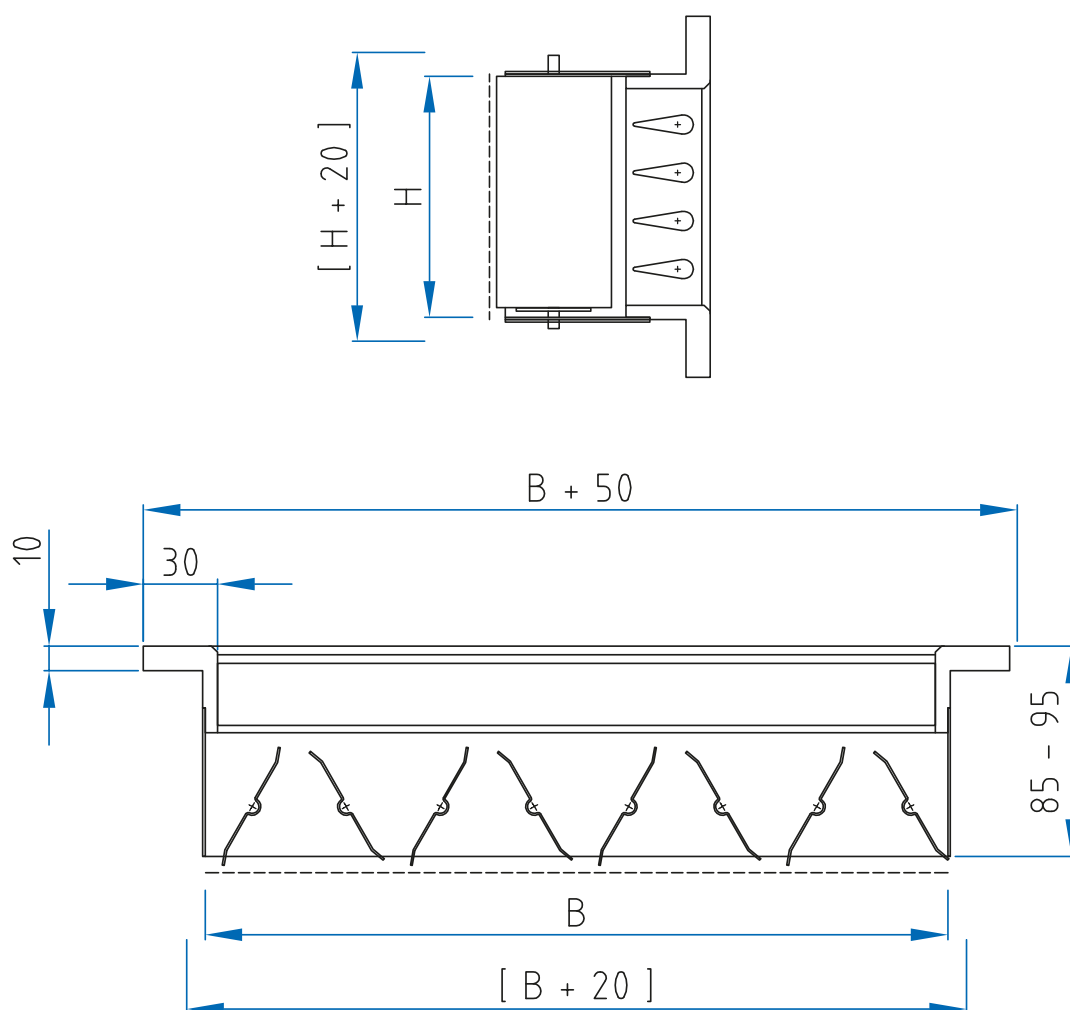
HG-130 HG-100 mit MKL-2 (gekoppelte gegenläufige Mengenregulierung)
