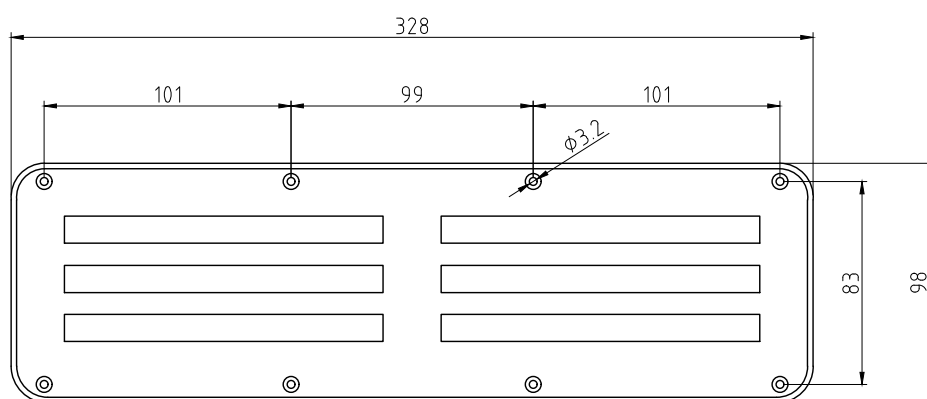
Ausschnittmaß 310x75 mm
